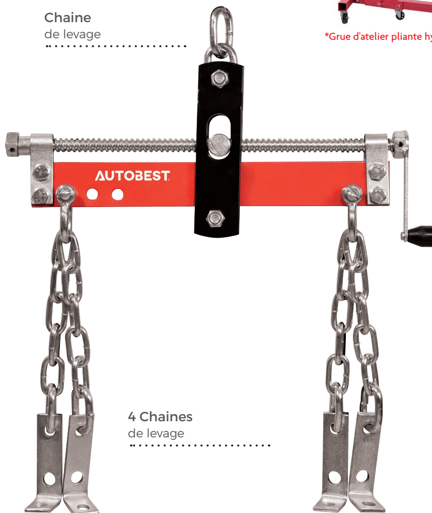
..... Manivelle d'équilibrage
